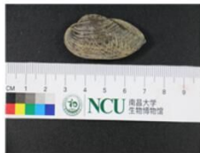
Unio persculpta
