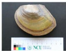
Anodonta woodiana
